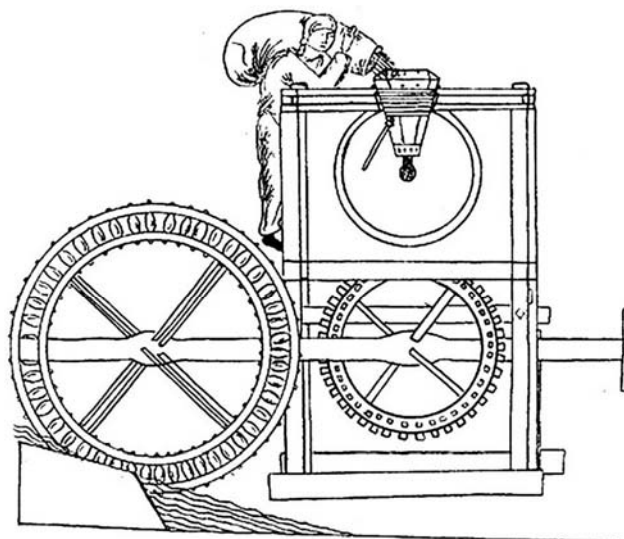
Moulin à eau, 1175-1185, d'après R. Pernoud, Hist. du Peuple français , t. I, pl. 24.
